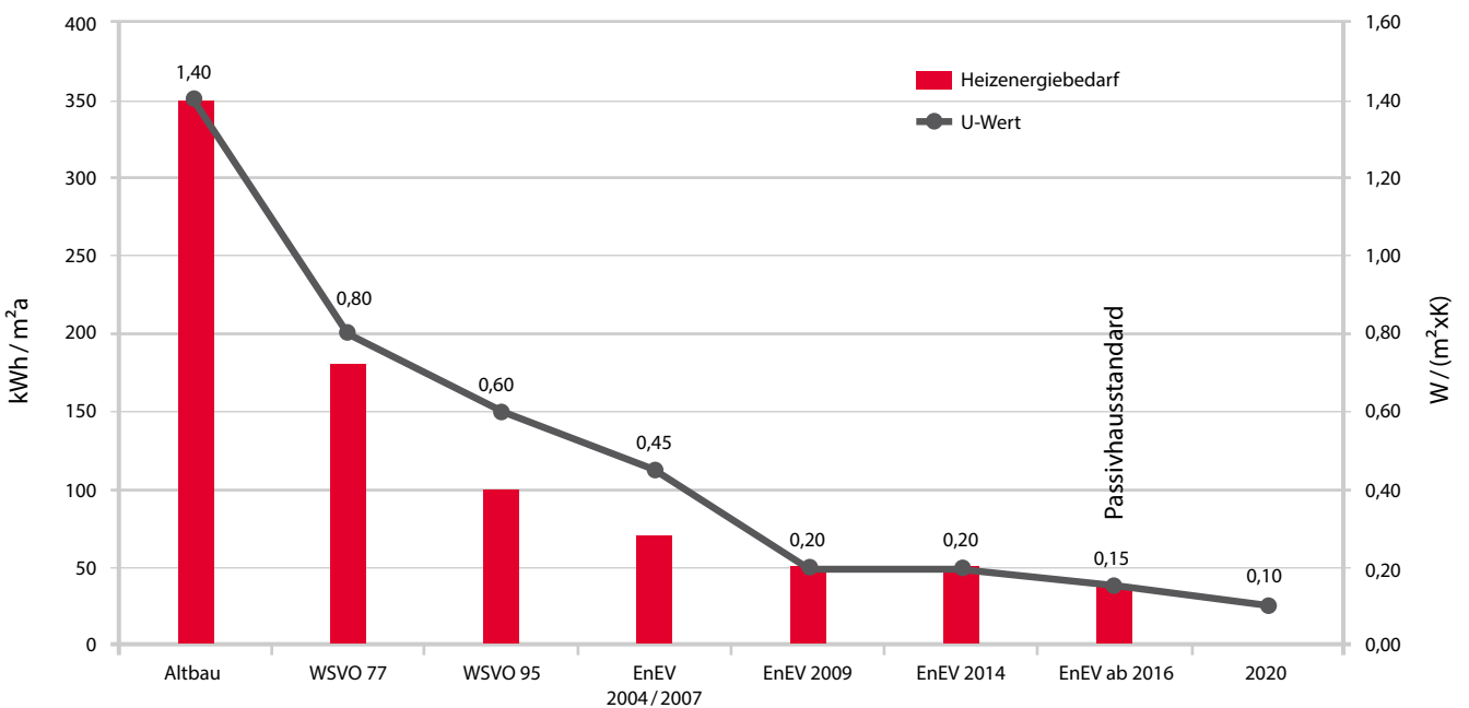
Entwicklung des Heizenergiebedarfs von Neubauten
