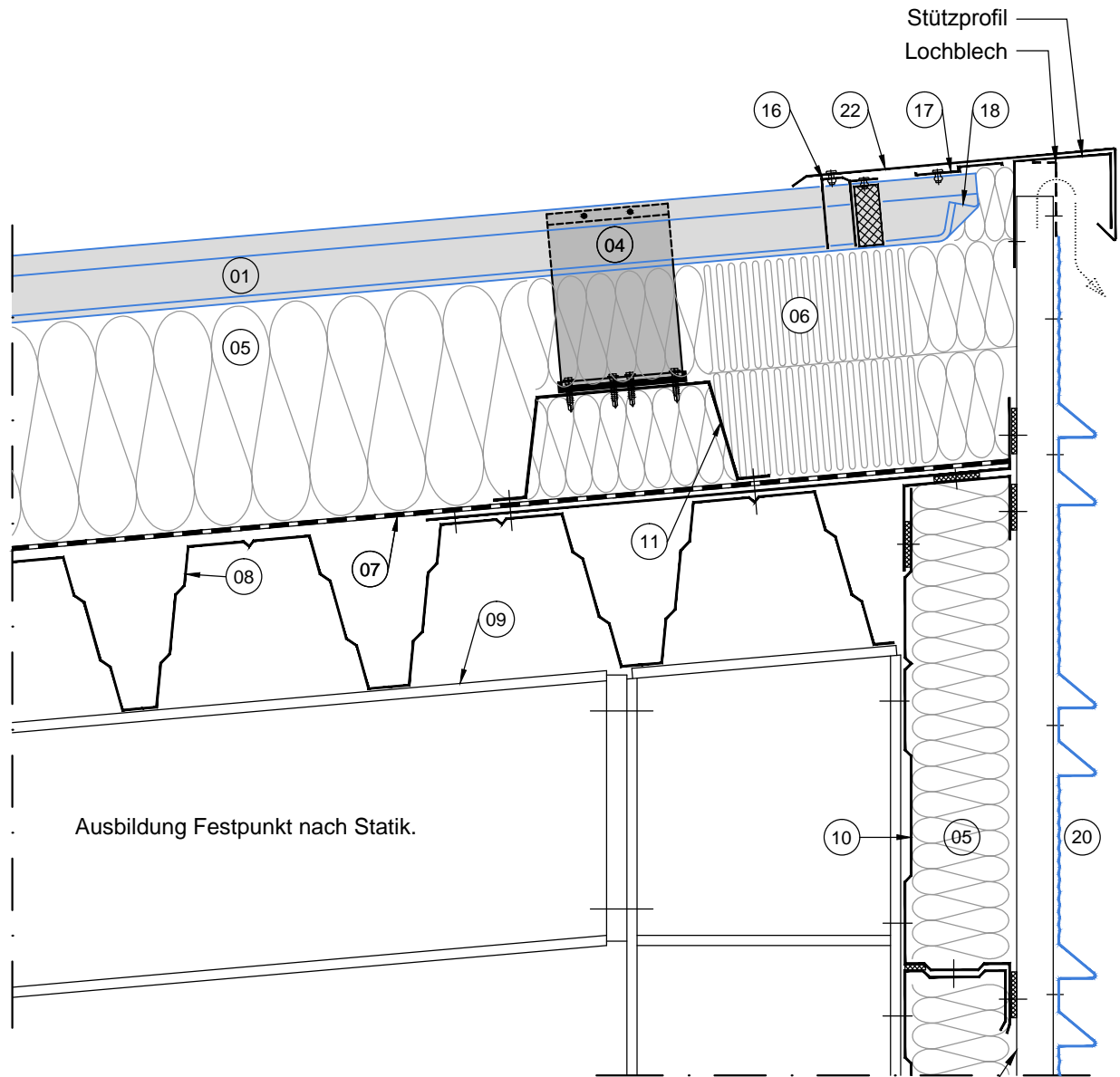
Unterkonstruktion für Kalzip TF und Aussteifung Kassettenprofile
