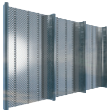
Kalzip® 65/500 P
